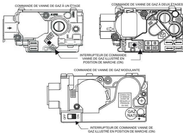
Figure 12 – Interrupteur de commande en position de marche (ON)
