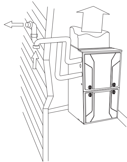
Figure 2 – Tuyaux d'évent extérieurs
